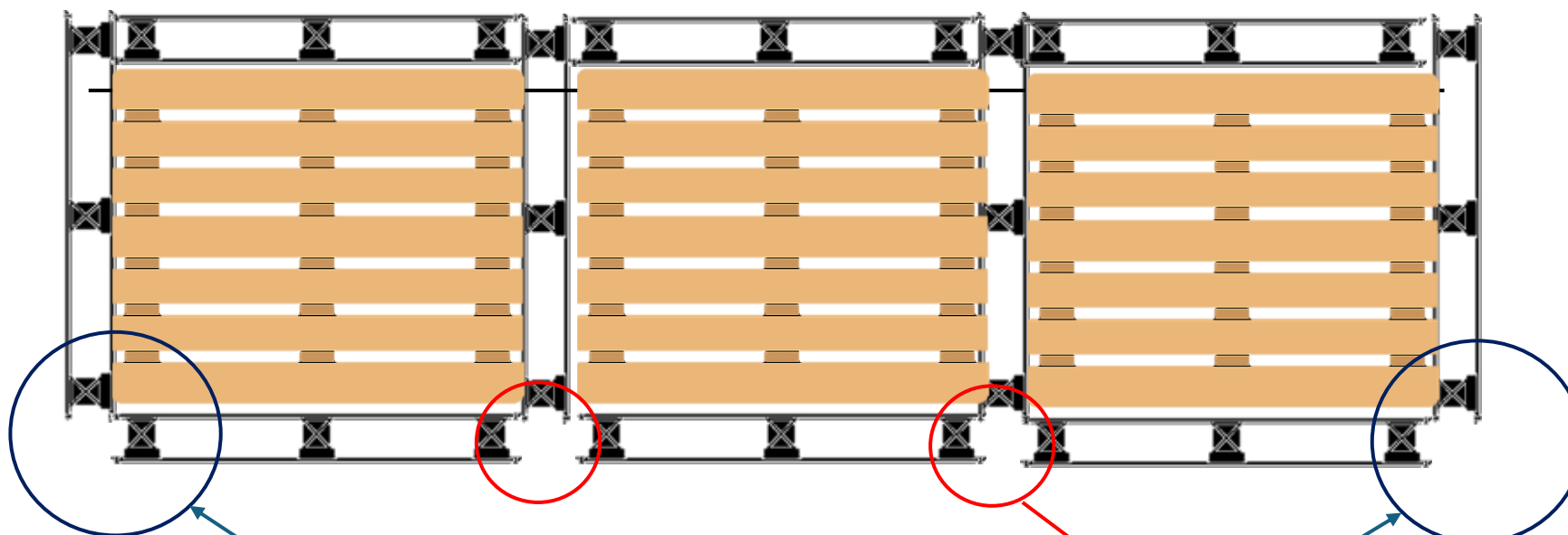
VISTA SUPERIOR
