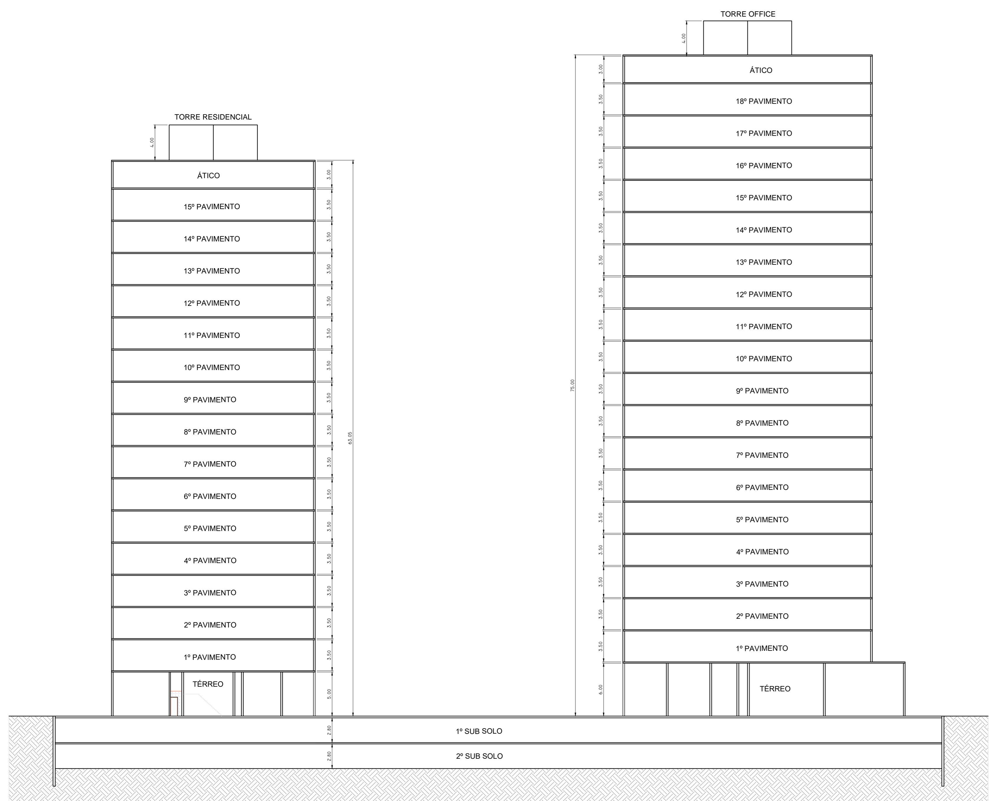
CORTE LONGITUDINAL A-A ESC. 1:250
