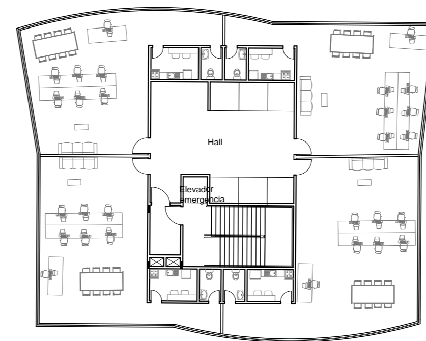
PLANTA DO PAV. TIPO (OFFICE) - 523,96m 2 ESC. 1:100
