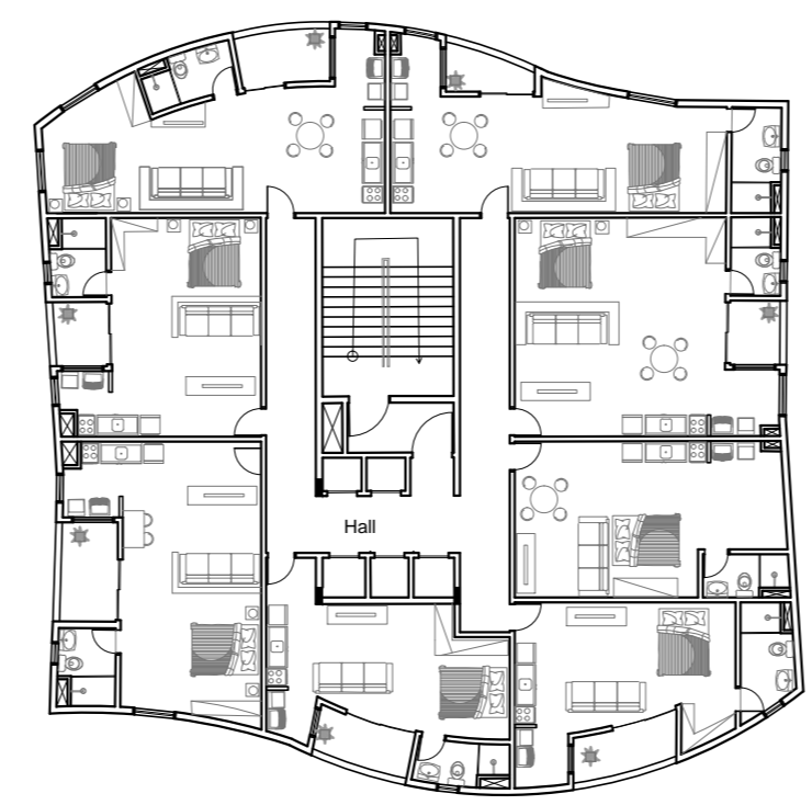
PLANTA DO PAV. TIPO (RESIDENCIAL - STUDIO) - 468m 2 ESC. 1:100
